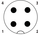
Pin ataması, M12 fiş, 4 pinli, A kodlu, fiş tarafının görünüşü
