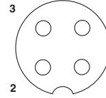
M12 socketin pin ataması, 4 pinli, A kodlu, dişi tarafın görünüşü
