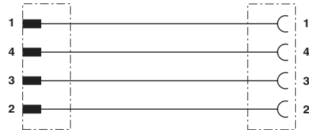
M12 fiş ve M12 socketin kontak ataması
