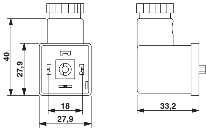
Boyutlu çizim
