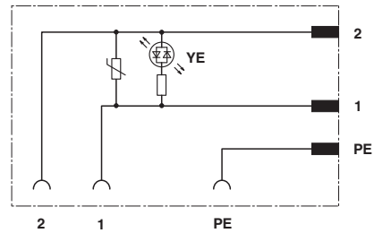
Devre şeması
