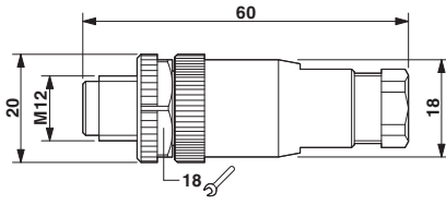
Boyutlu çizim
