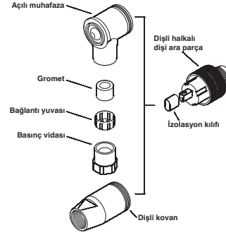
Şematik diyagram
